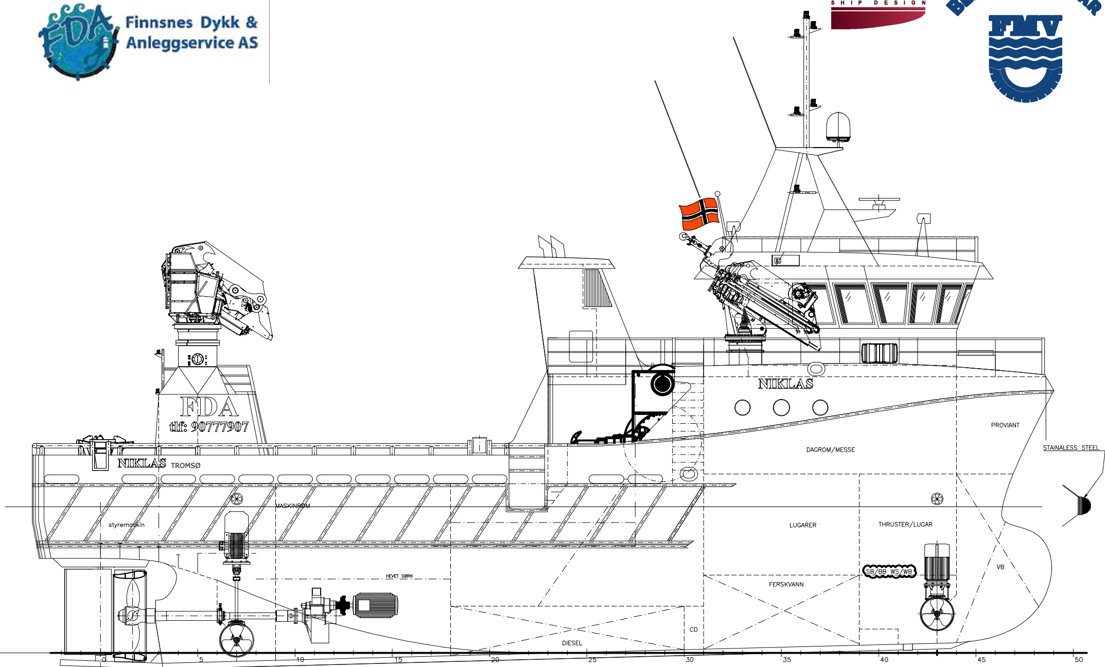
PROFIL SB
