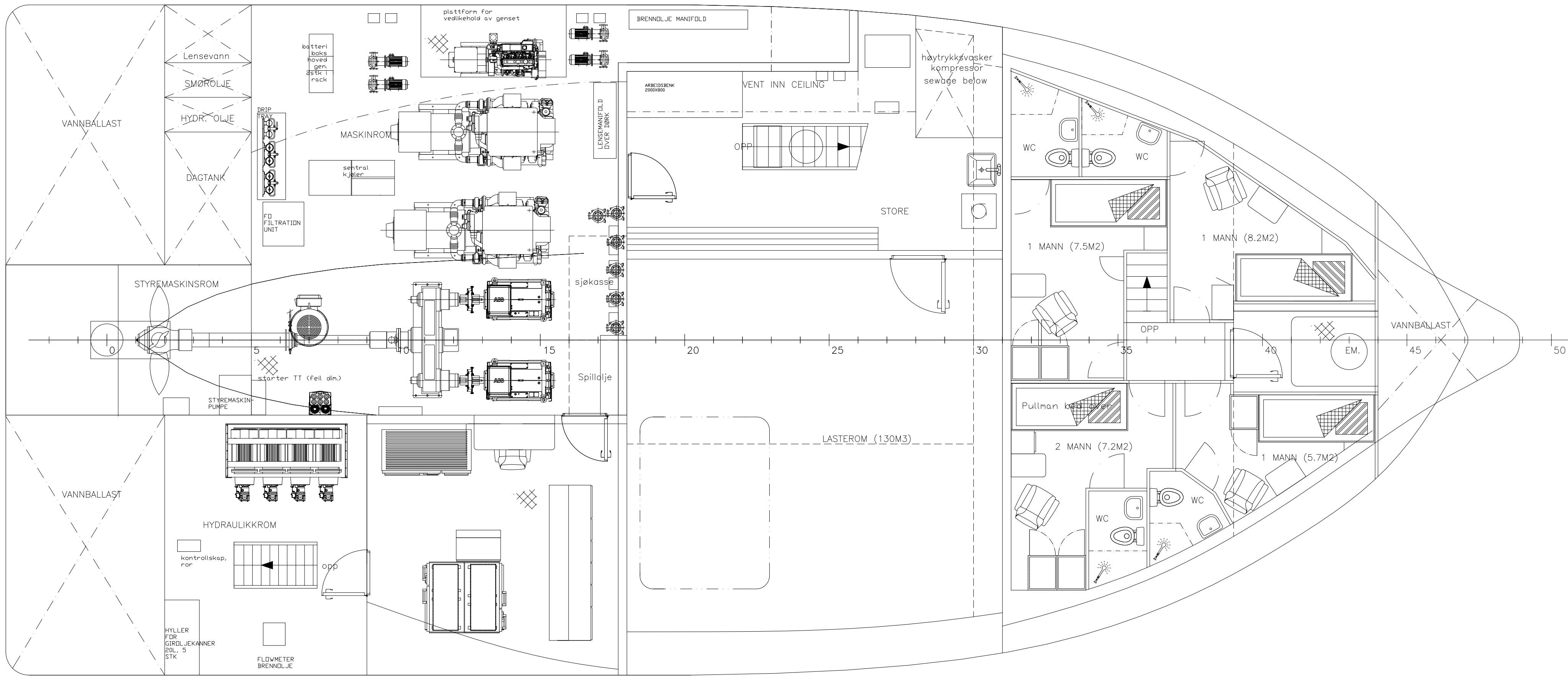
UNDER HOVEDDEKK
