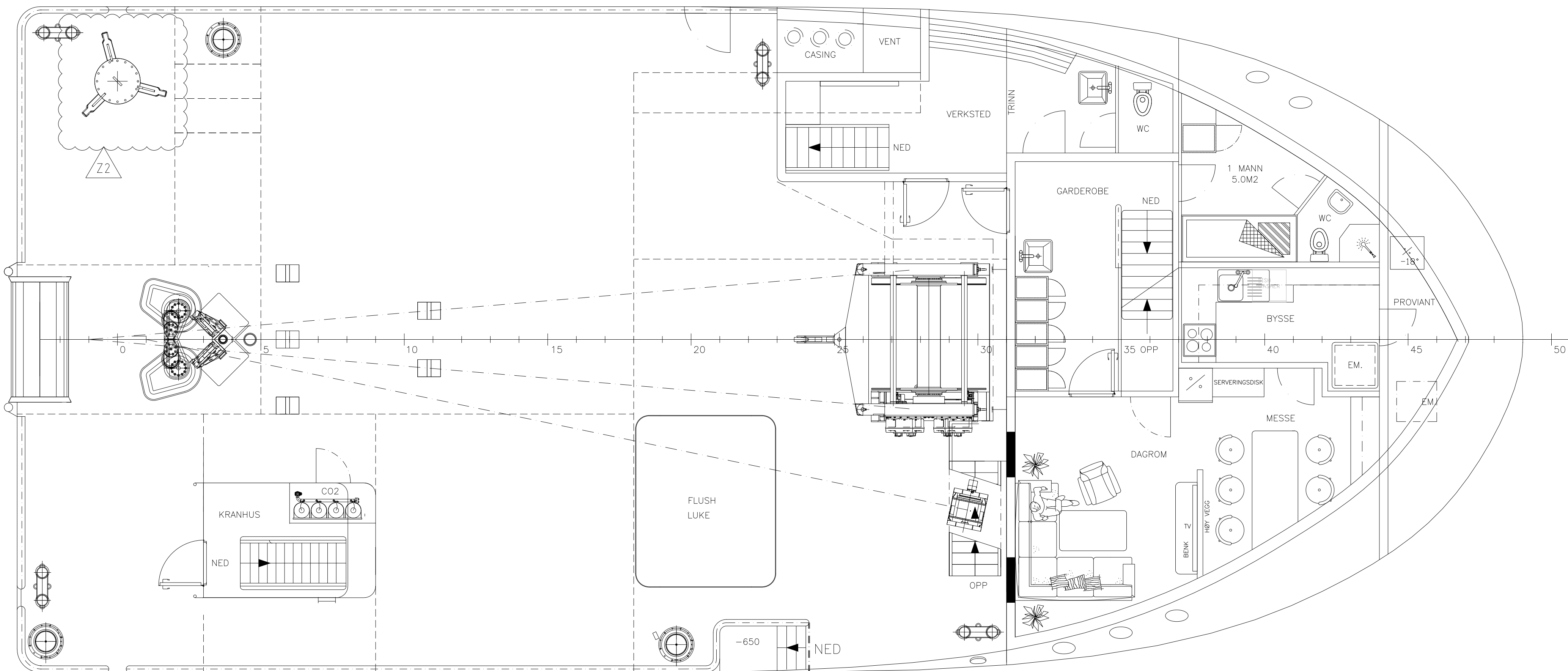
HOVEDDEKK
