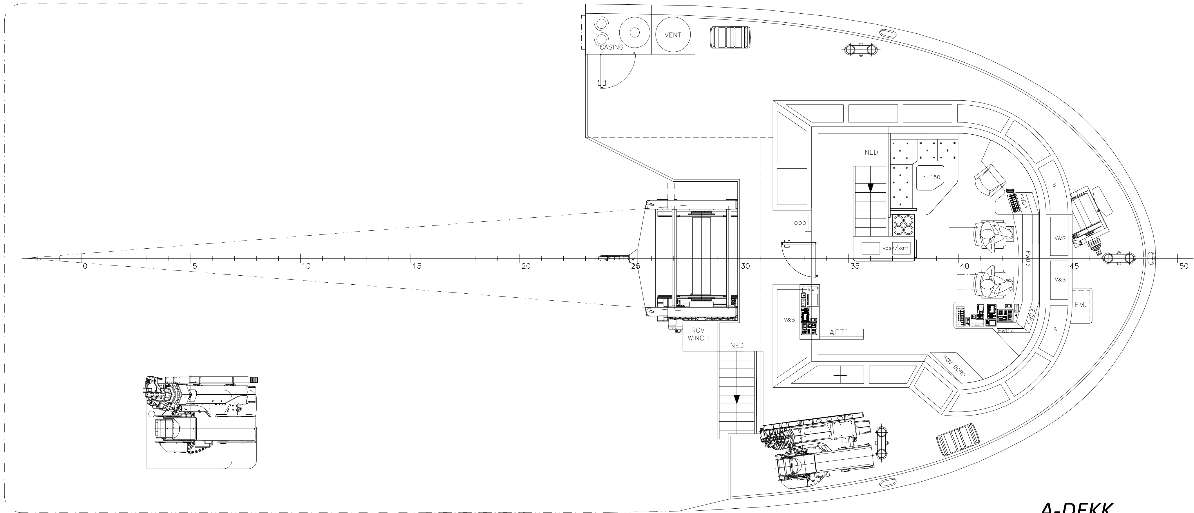
A-DEKK
